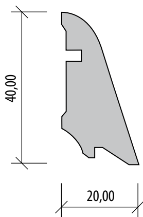
Lišty Hoco 554 UM
