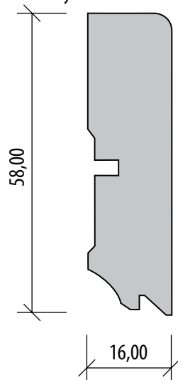
Lišty Hoco 631 UM CUBE
